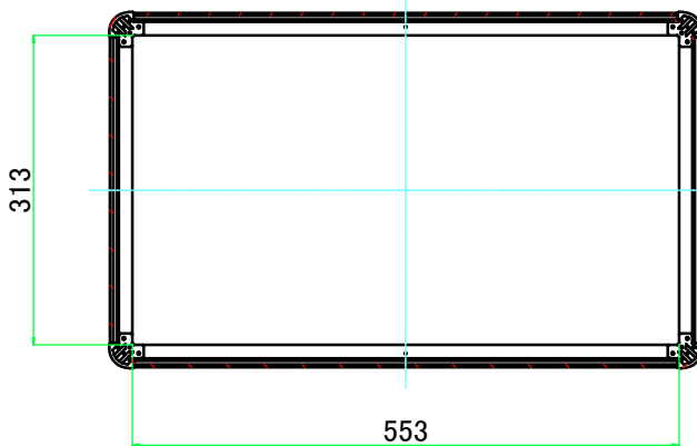
C-C ( 1 : 8.5 )
